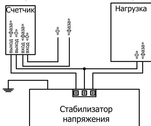
Рекомендуемая схема подключения стабилизатора к сети
